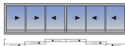
Εξάφυλλο επάλληλο φιλτρά συρόμενο (φιλτρά έξω)
