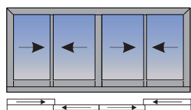
Τετράφυλλο επάλληλο φιλτρά συρόμενο (φιλτρά μέσα)
