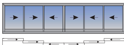
Εξάφυλλο επάλληλο φιλτρά συρόμενο (φιλτρά μέσα)
